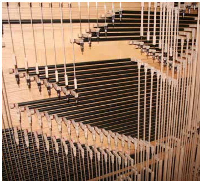
Notranjost orgel - razdelilna deska za igralno mehaniko
